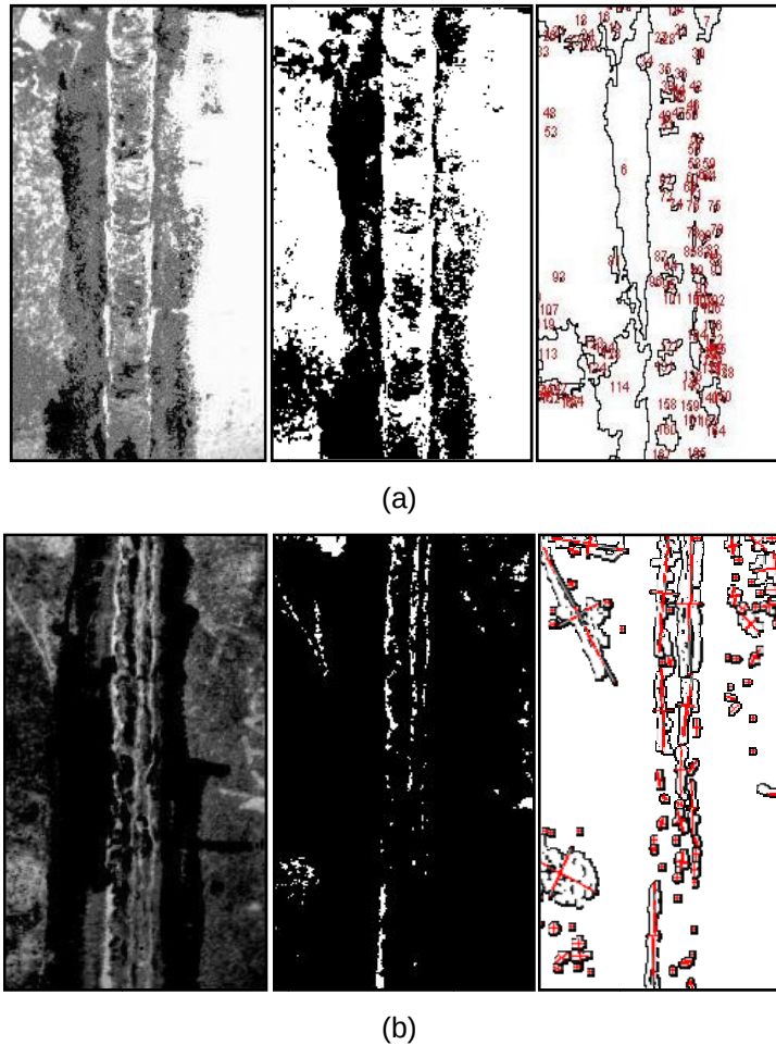
Fig. 5. Proceso de segmentación y operaciones morfológicas de las probetas (a) EO – 26 y (b) EO – 13
