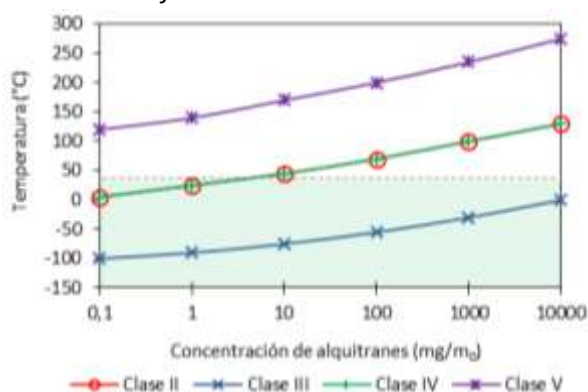
Fig 1. Punto de rocío de las clases de alquitrantes 2-5, en función de la temperatura y concentración. Fuente: Tomado y adaptado de [8]
