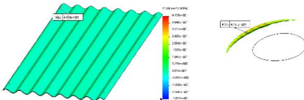
Fig 5. Distribución de tensiones principales en la plancha del nuevo material compuesto
