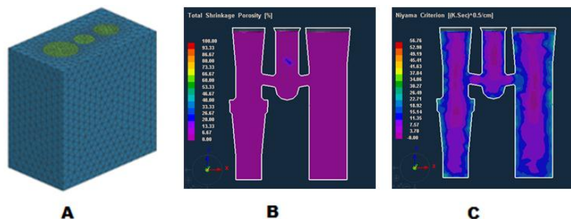
Fig 4. Imagen en 3D del molde mallado (A), resultados de la porosidad (B) y del criterio de Niyama (C). Fuente: Autores
