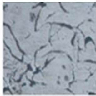
Fig 3. Muestra de la micro estructura del material para el molde obtenida a 200X. Fuente: autores
