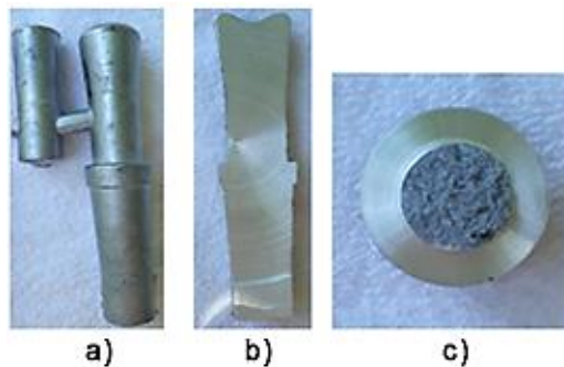
Fig. 8. Semiproducto fundido: a), semiproducto seccionado, b), parte de pieza fracturada c). Fuente: autores
