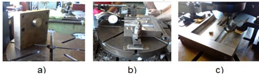
Fig. 7. Dispositivo para el centrado: a), instalación en la mesa divisora, b) elaboración de alimentadores, c). Fuente: autores
